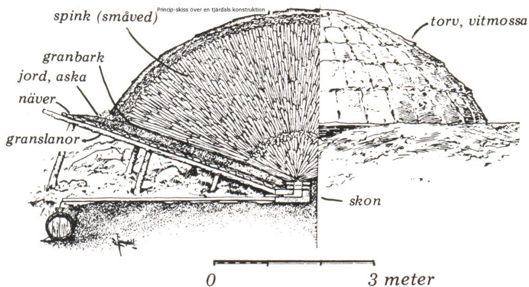
Principskiss för hur en tjärdal är uppbyggd.
